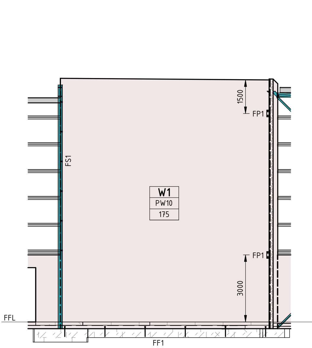
SECTION 1B SCALE 1 : 100
